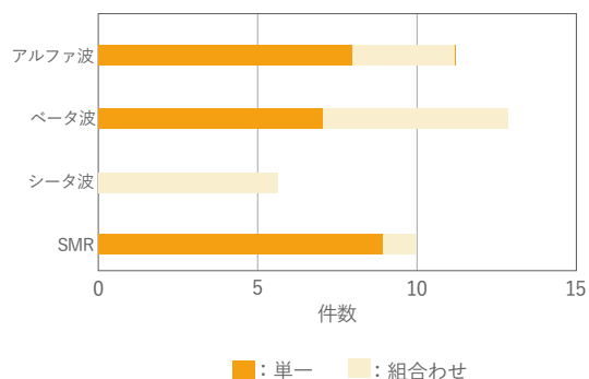
(C) NFT に用いられている脳波成分
