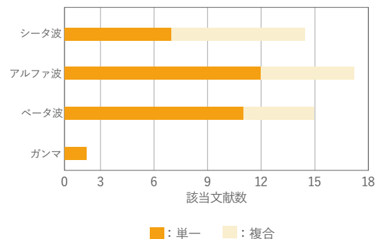
(C) NFT 対象周波数帯
