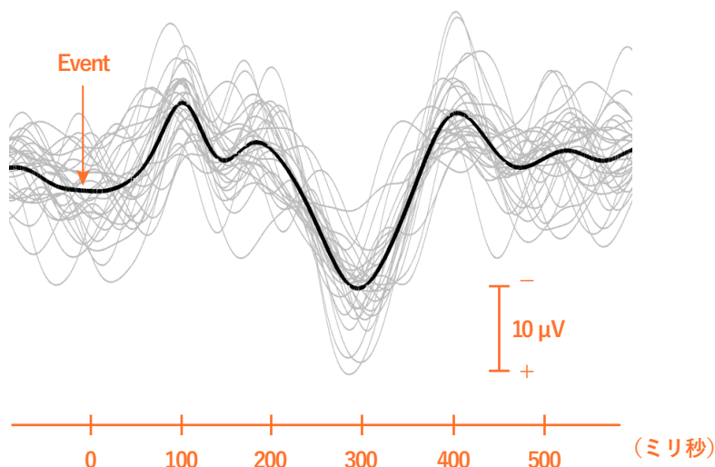
図2.聴覚刺激に対する事象関連電位の例。聴覚刺激という1回の事象に対して複数のピークが現れます。灰色の細線は事象1回ごとの波形、黒色の太線は事象30回分の平均波形を表します。平均化により、自発脳波の揺らぎやノイズなどの影響を抑えて事象関連電位の成分を検出できます。
