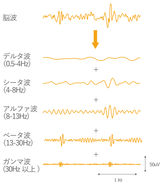
図 1. 脳波計で記録される脳波の様子。脳波はそのリズムの速さを示す周波数(Hz)によって分類されます。
