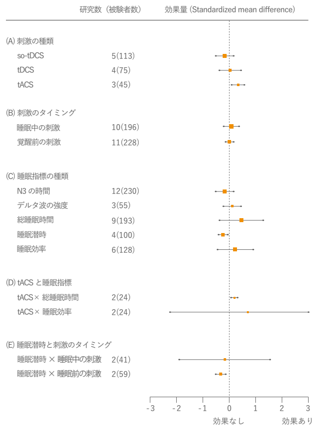
図1. 有効性の評価結果。(A) 刺激法ごとの効果。(B) 刺激のタイミングごとの効果。(C) 睡眠指標ごとの効果。(D) tACS による睡眠指標ごとの効果。(E) 睡眠潜時に対する刺激タイミングの効果。
