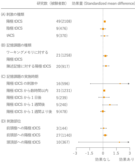
図 1. 有効性の評価結果。(A) 刺激法ごとの効果。(B) 記憶課題ごとの陽極 tDCS の効果。(C) 記憶課題の実施時期ごとの陽極 tDCS の効果。(D) 刺激部位ごとの陽極 tDCS の効果。
